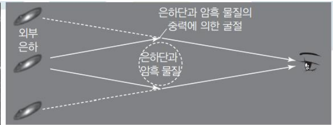
은하단과 암흑 물질에 의한 중력 렌즈 현상으로 외부 은하가 왜곡되어 보이는 모습
