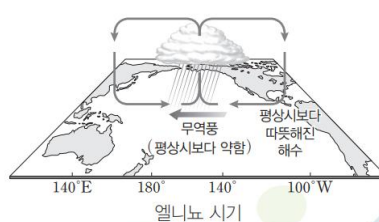
엘니뇨와 라니냐 시기의 워커 순환
